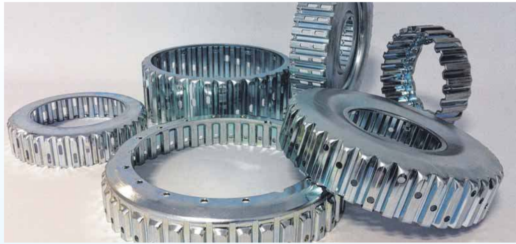
Metallische Bauteile eines Getriebes werden umformtechnisch hergestellt.
